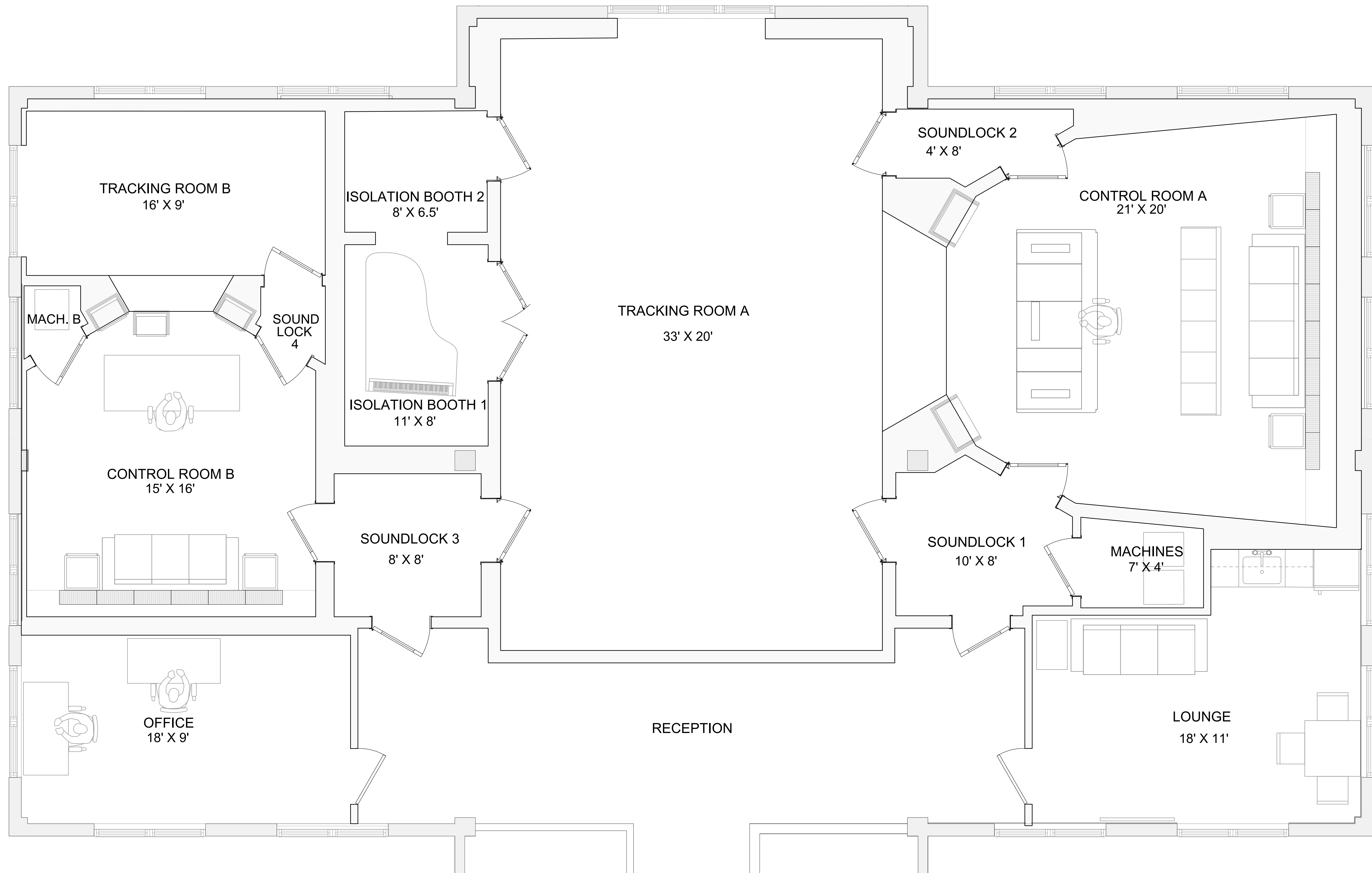
1 AC STUDIO LAYOUT SCALE: 3/8"=1'-0"
